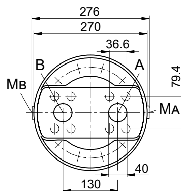
Detail Y
