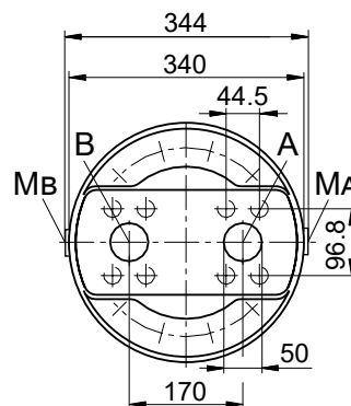
Detail Y
