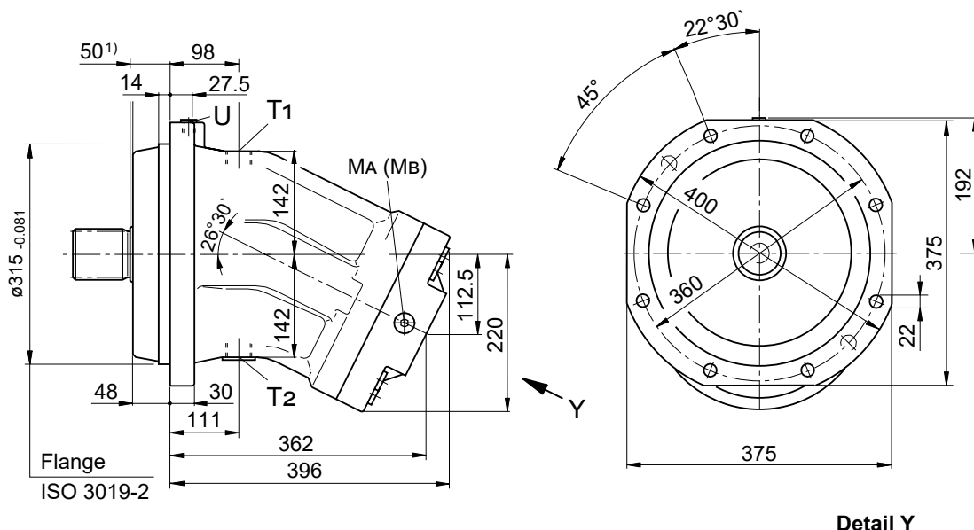
Detail Y
