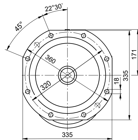
Detail Y
